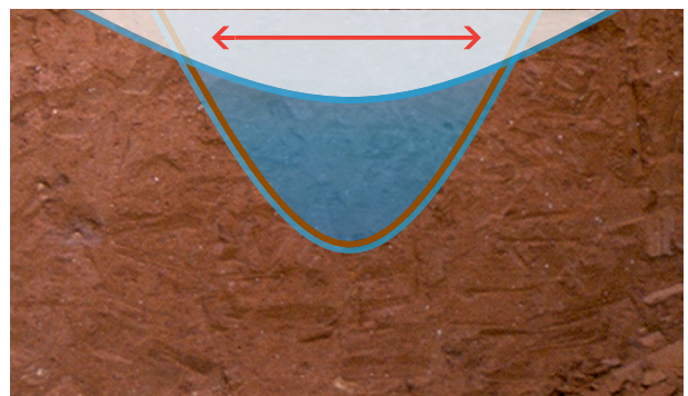
SUOLI ARGILLOSI
