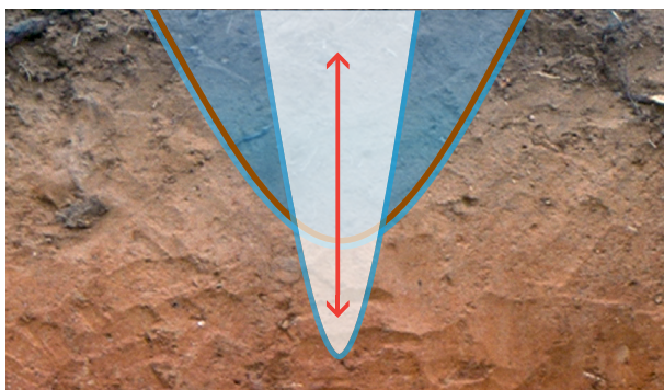
SUOLI SABBIOSI
